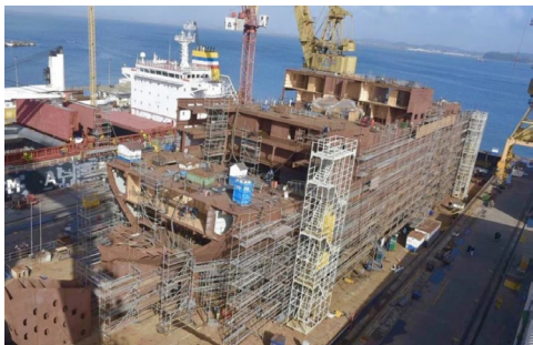
Rompehielo AGB 46 "Almirante Óscar Viel": Construcción en Astillero ASMAR (T), y navegación en las aguas del Mar de Weddell, aprobando sus pruebas de hielo de verano. (Fuente: Armada de Chile)
